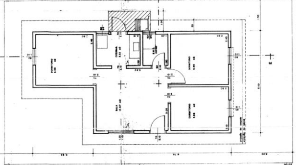
PLANTA ESC. 1:50 - BU1-3-42 A CONSTRUIR - 41,86 m²
