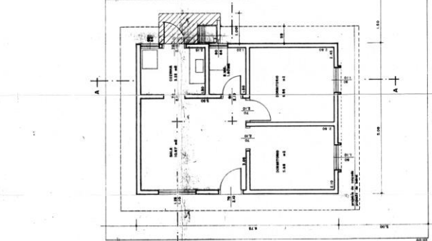
PLANTA ESC. 1:50 - BU1-2-34 A CONSTRUIR - 33,75 m²
