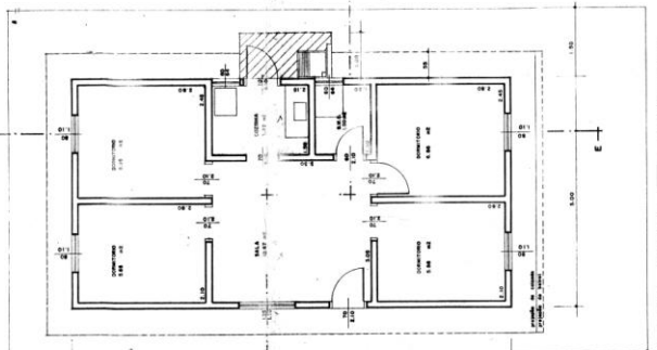
PLANTA ESC. 1:50 - BU1-4-49 A CONSTRUIR - 68,20 m²
